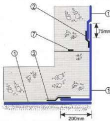
Oszlop részletterv
