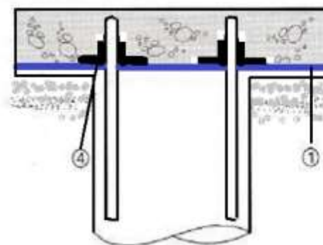
Oszlop részletterv
